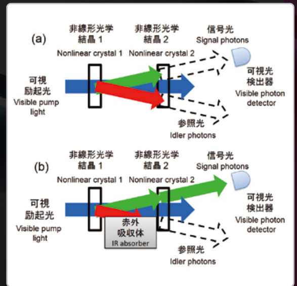
赤外量子吸収分光のイメージ Image of infrared quantum absorption spectroscopy
