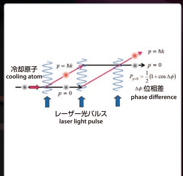
光パルス型原子干渉計 Light pulse-based atomic interferometer
