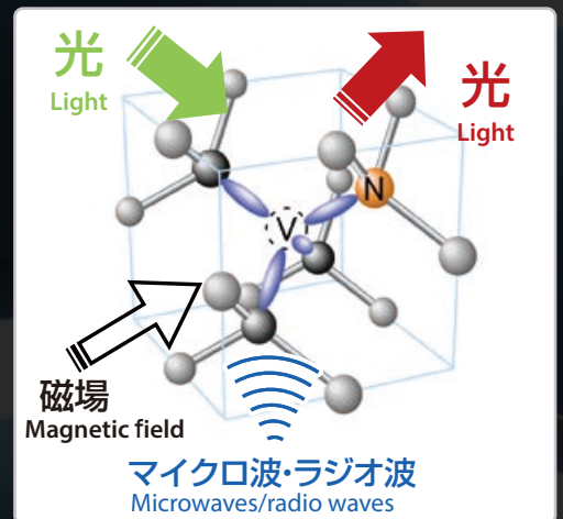
ダイヤモンドNVセンタ Diamond NV center
