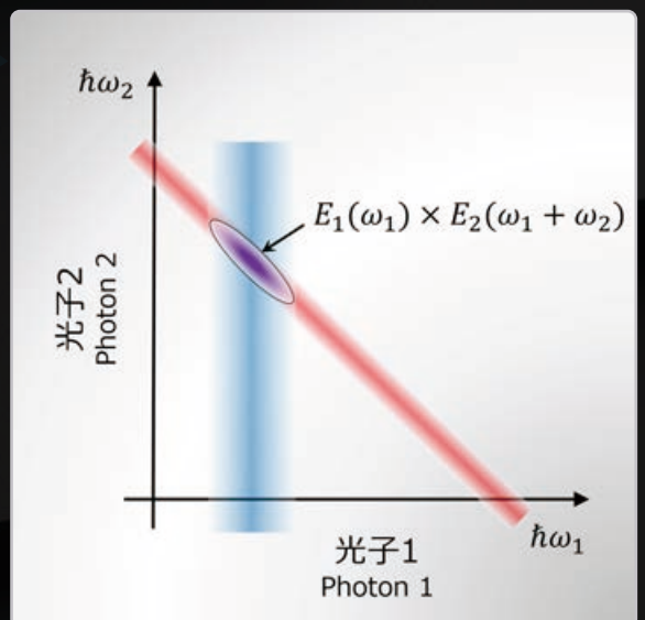
二次元量子分光の原理 Principles of 2D quantum spectroscopy
