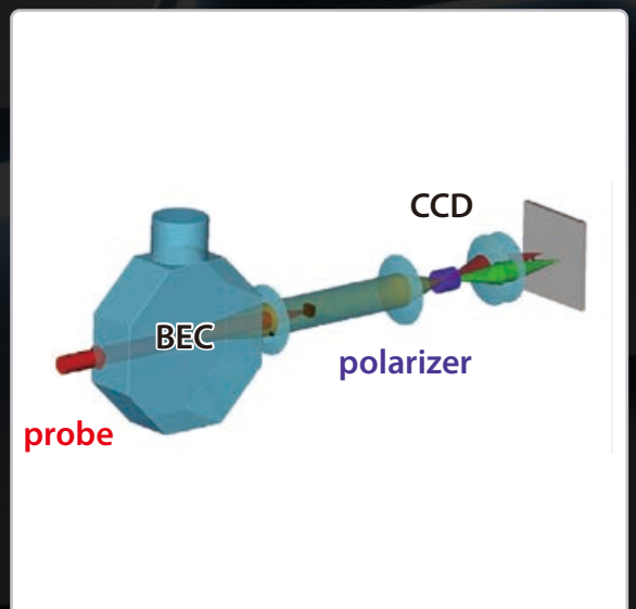
ボース・アインシュタイン凝縮体空間磁力計の模式図 Schematics of Bose-Einstein condensate spatial magnetometer
